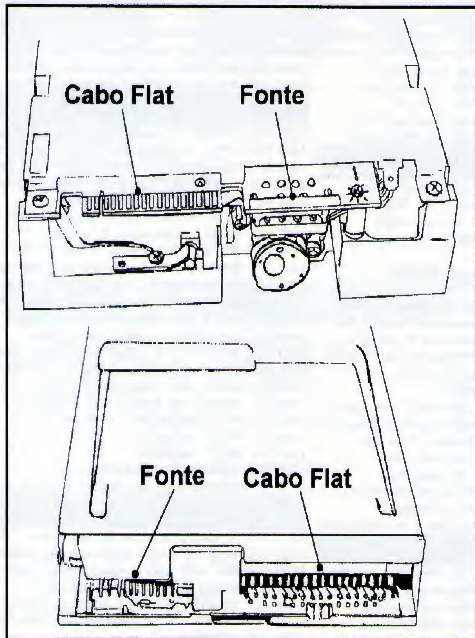
Figura 19 - conexões na parte traseira dos drives
